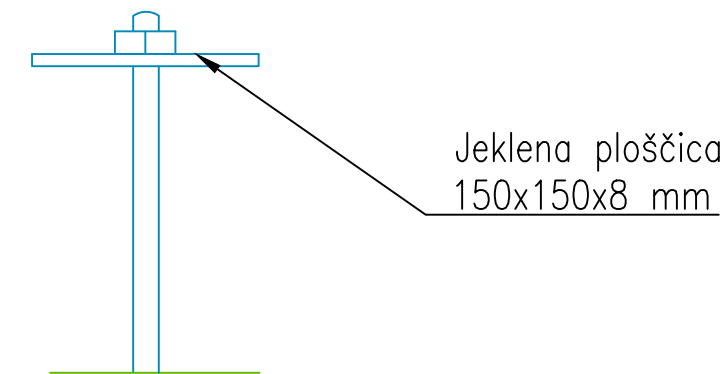
PALIČNO SIDRO S PLOŠČICO IN MATICO
