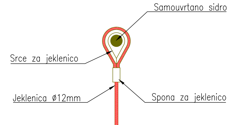
PENTLJA JEKLENICE Z NOTRANJIM JEKLENIM PRSTANOM
