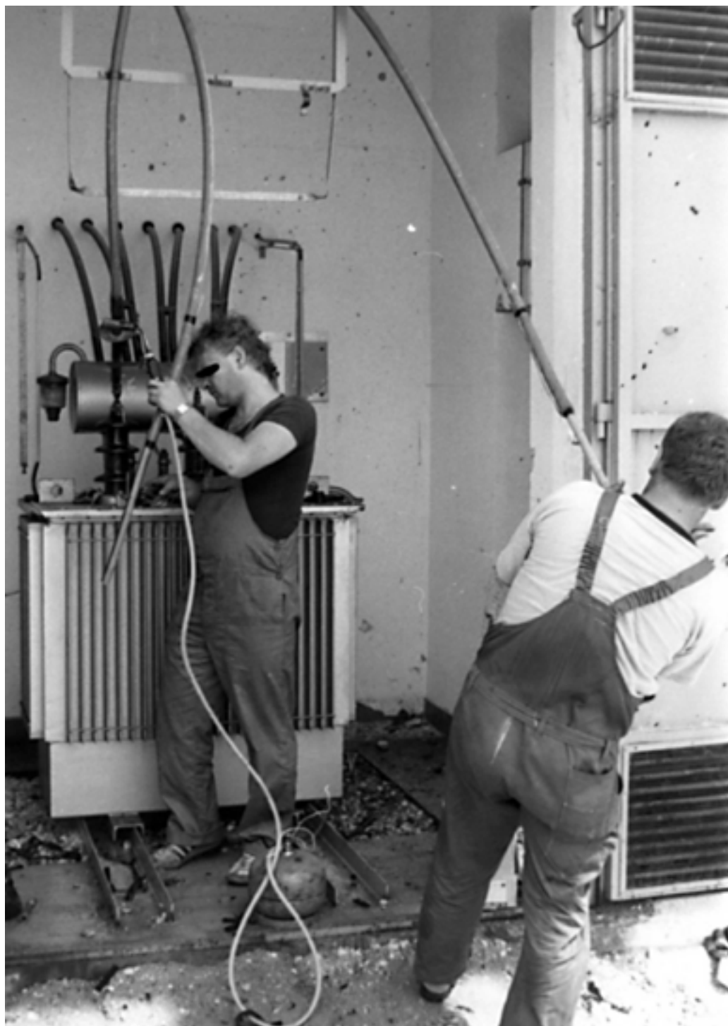
Slika 111: Ekipa je opravila demontažo poškodovanih transformatorjev: skrajšala kabel povezave, izdelala nove končnike in montirala nove transformatorje. Na fotografiji električarja pri delu na Krvavcu, 2. julija 1991. Vir: Arhiv dr. Draga Paplerja
