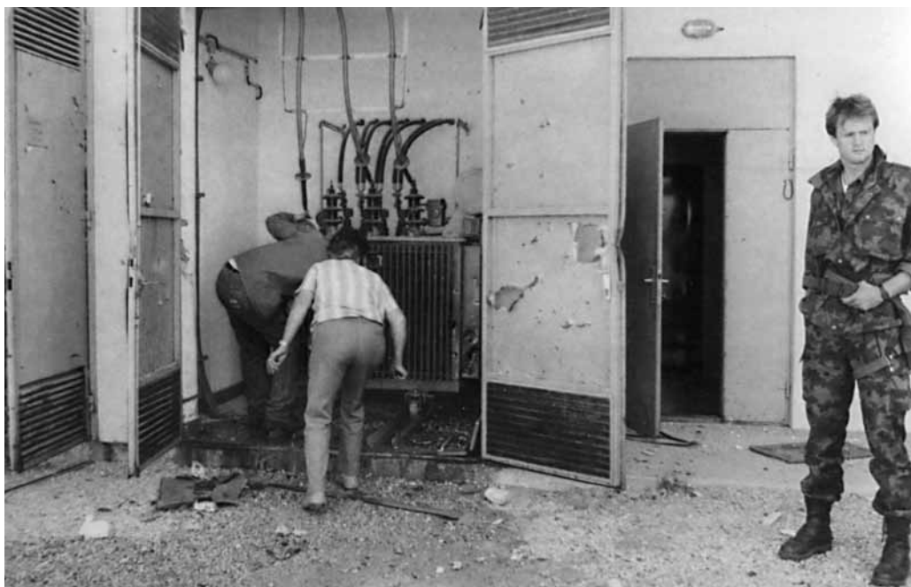
Slika 112: Prvi transformator je bil popolnoma uničen, iz njega je odtekalo olje, drugi je imel uničena hladilna rebra Vir: Arhiv dr. Draga Paplerja
