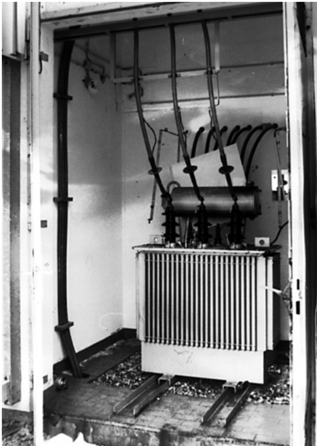
Slika 108: Transformatorju je izteklo transformatorsko olje Vir: Arhiv dr. Draga Paplerja
